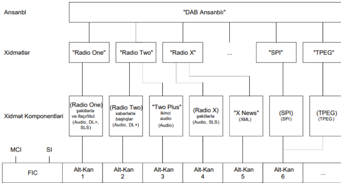
Şəkil 18: DAB xidmət strukturunun nümunəsi
