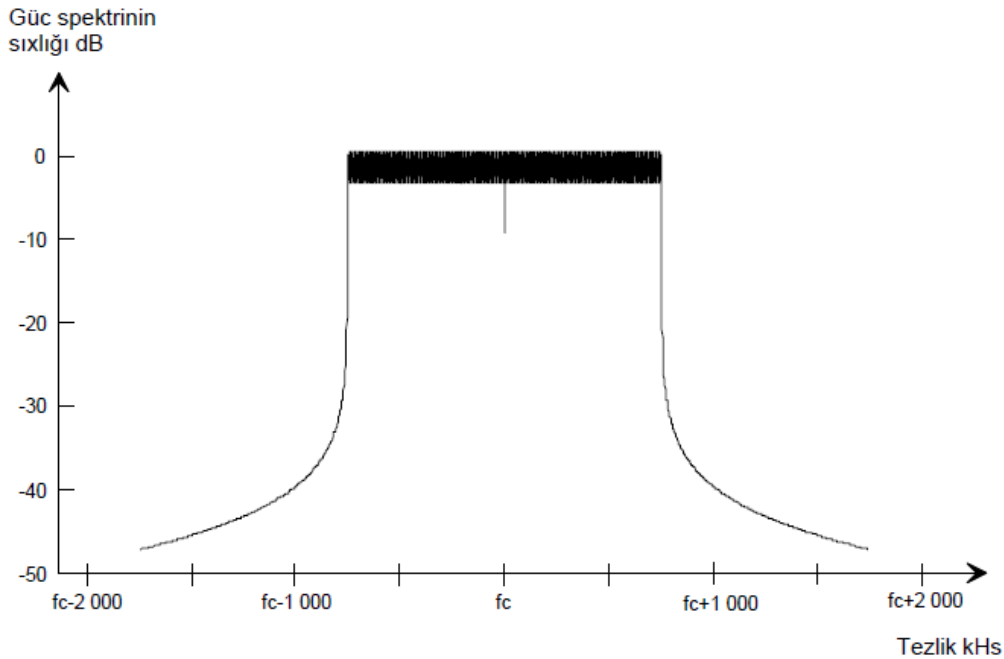
Şəkil 65: I ötürmə rejimi üçün nəzəri DAB ötürmə siqnal spektri
