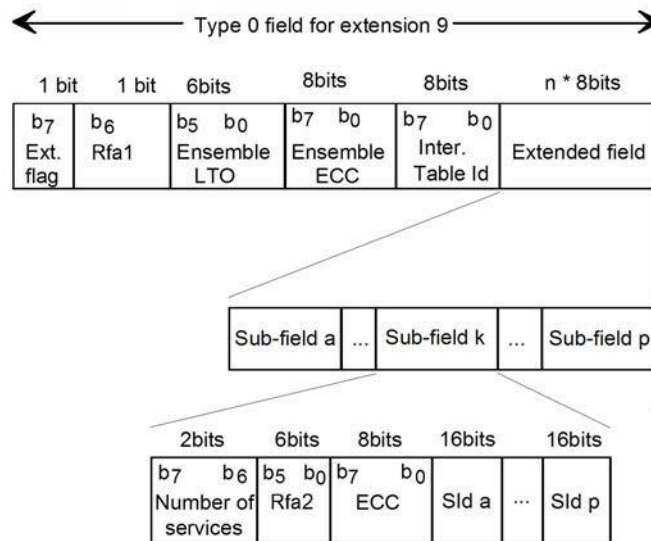
Şəkil 39: Ölkə sahəsinin strukturu
