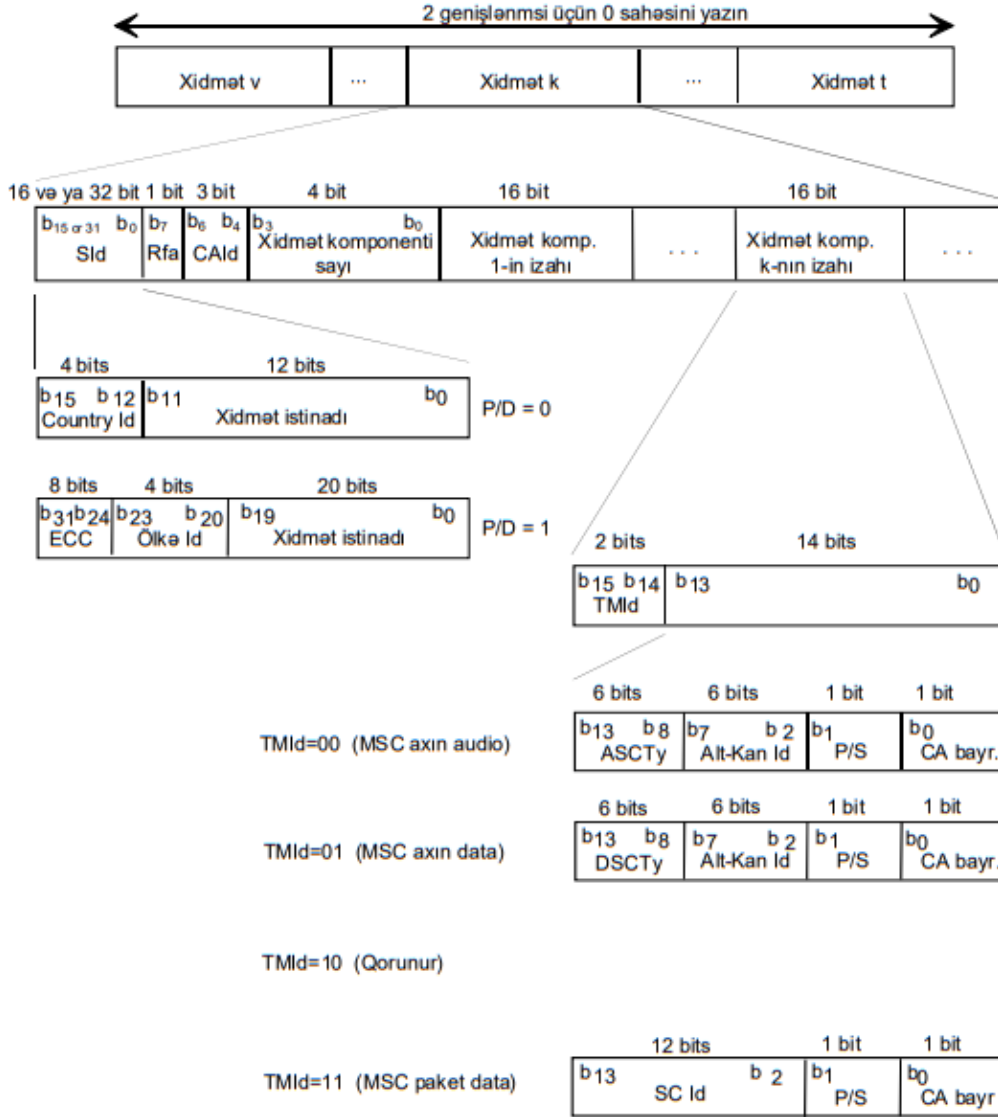
Şəkil 21: Xidmətin təşkili sahəsinin strukturu
