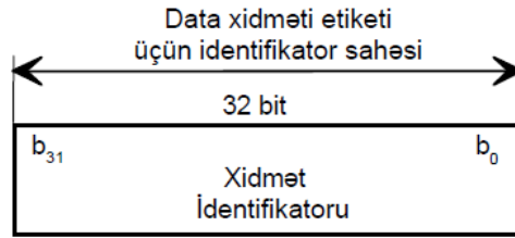
Şəkil 50: Data xidmət etiketi üçün İdentifikator sahəsinin strukturunu
