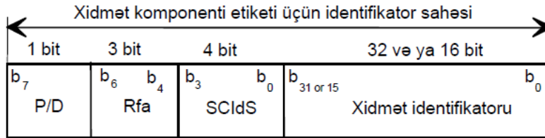
Şəkil 51: Xidmət komponenti etiketi üçün İdentifikator sahəsinin strukturunu
