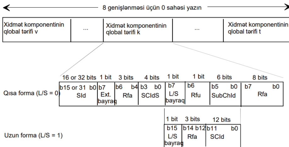
Şəkil 24: Xidmət komponentinin qlobal tərifi sahəsinin strukturu
