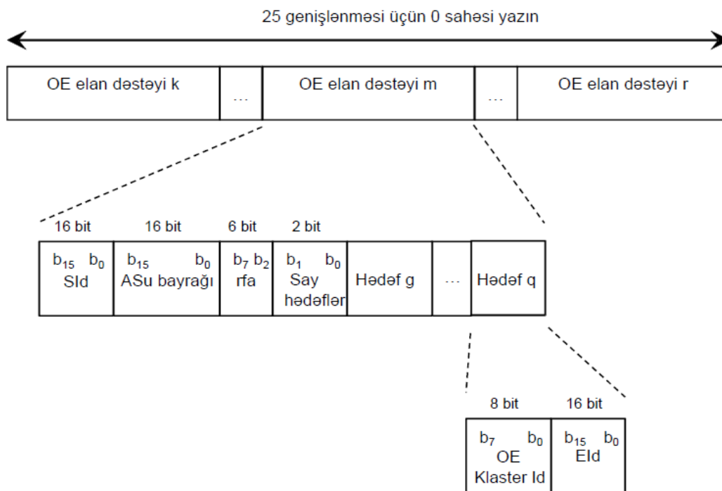
Şəkil 44: Digər ansamblın anons dəstəyi sahəsinin strukturu
