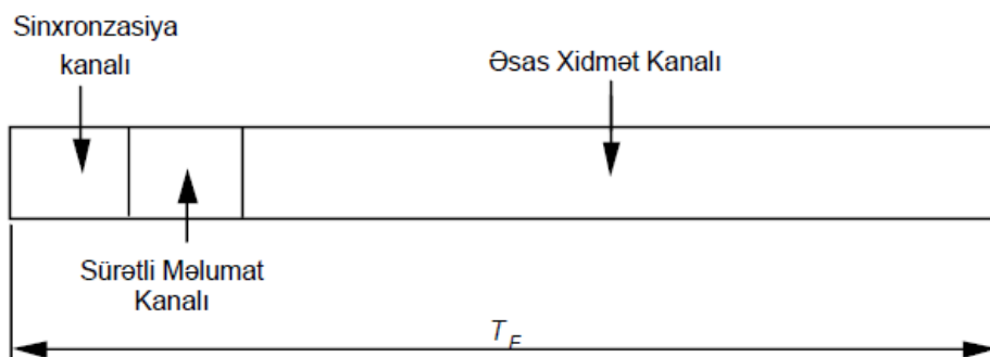
Şəkil 60: Transmissiya çərçivəsinin quruluşu
