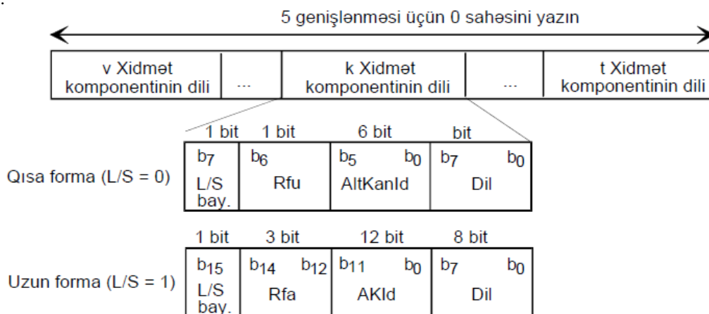
Şəkil 37: Xidmət komponenti dil sahəsinin strukturunu
